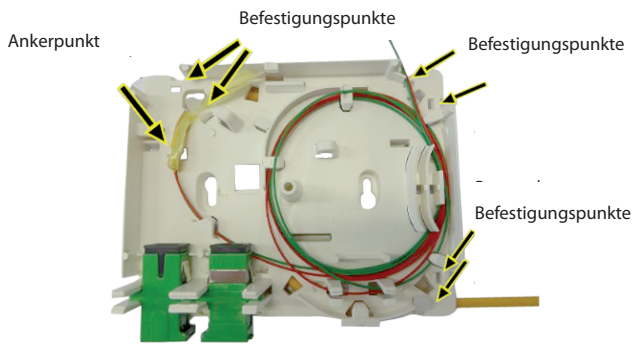
Unterbringung der Glasfaser im Inneren der Box
