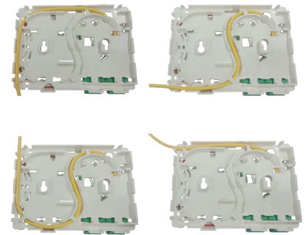
Kabeldurchführung
